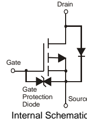
SOT-23
